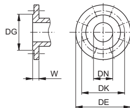
Flanges EN 1092-2
