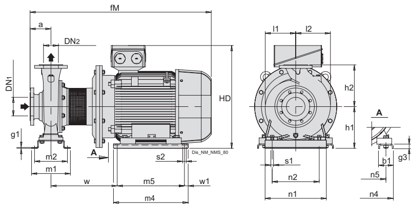
Flanges EN 1092-2
